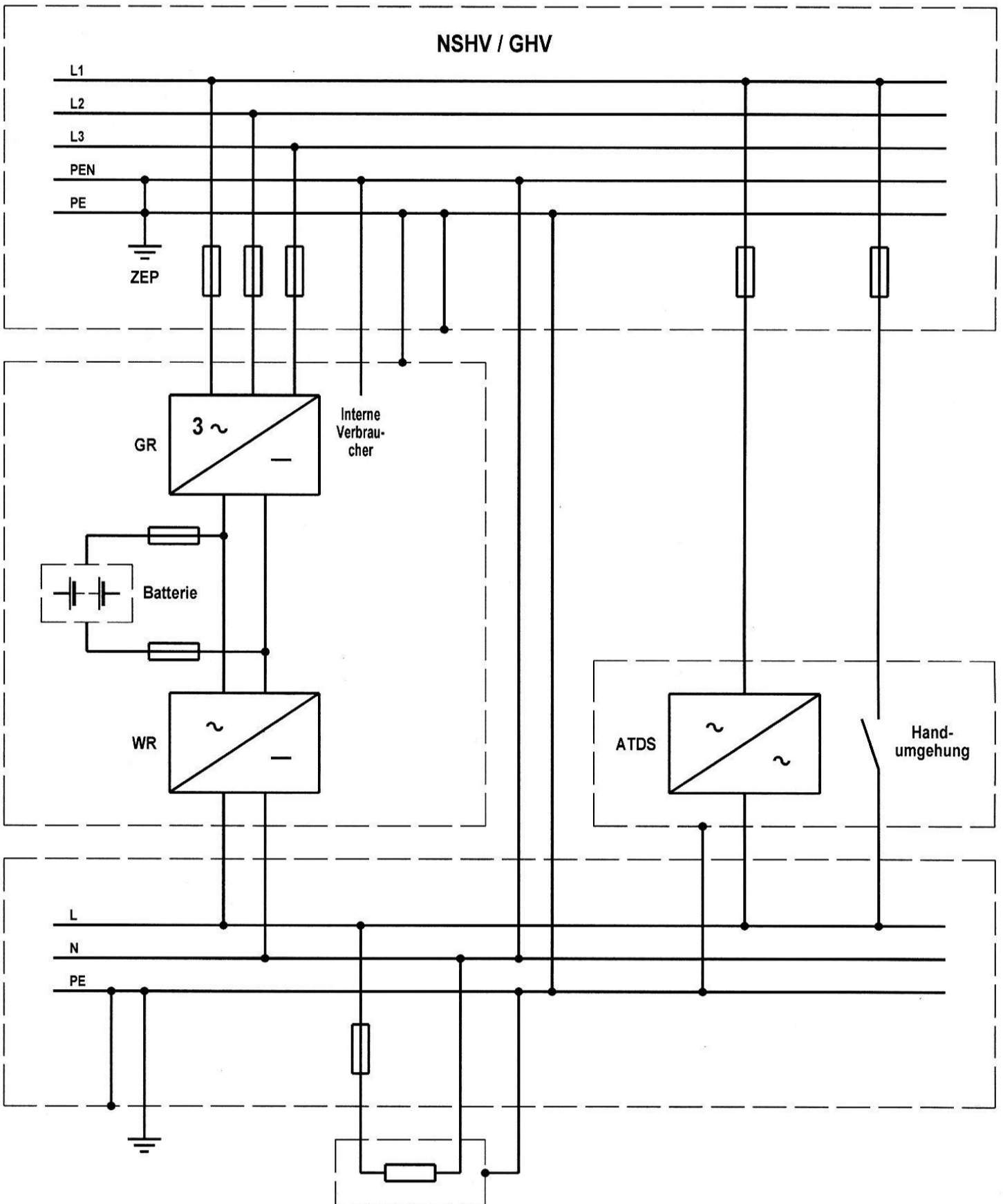
Bild 1: Batteriegestützte Stromversorgung im TN-S-System
